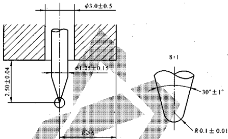
图1 D型邵氏硬度计压针几何形状
