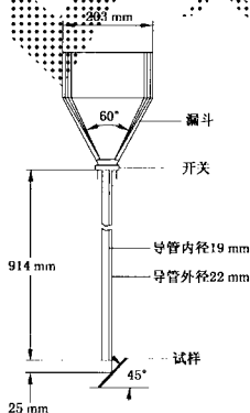
图 A.1 耐磨性仪器结构示意图
