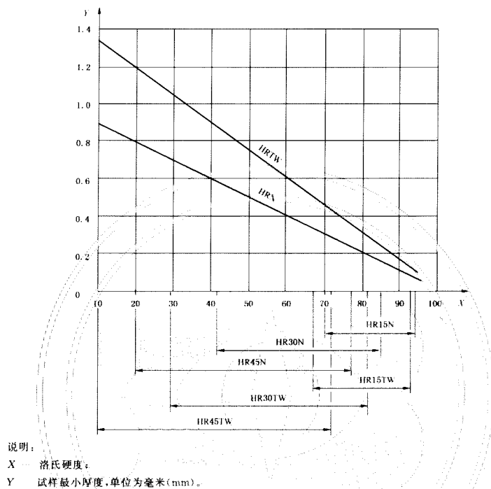
图 B.3 表面洛氏硬度试验(N和T标尺)
