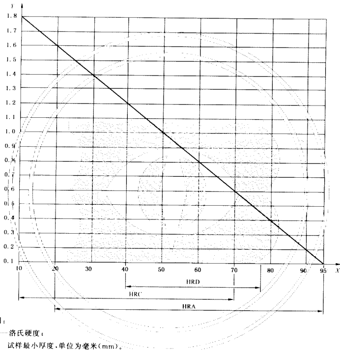
图 B.1 用金刚石圆锥压头试验(A、C、和 D 标尺)
