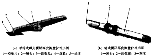
图 2 磁力式覆层厚度测量仪外形图
