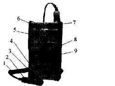
(b) 指针式覆层厚度测量仪外形图
