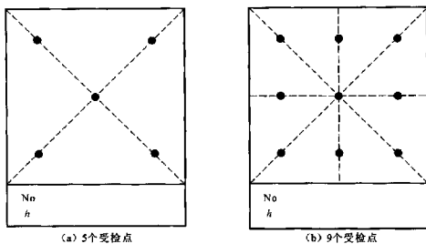
图3 校准厚度片的测量位置和测量点数示意图
